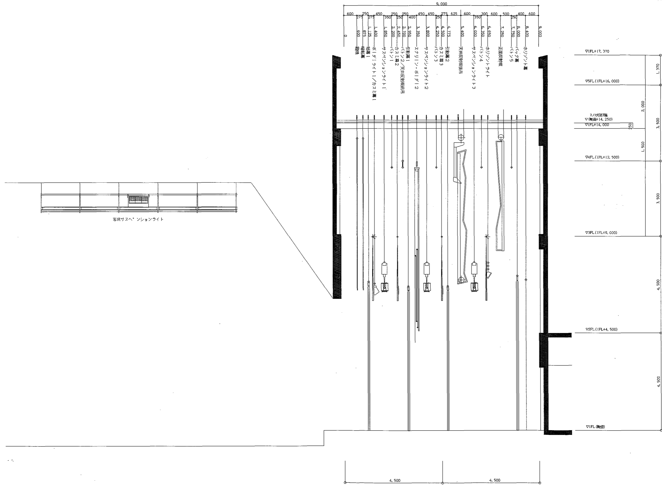
始良市文化会館小ホール舞台断面図 A3 1/100
